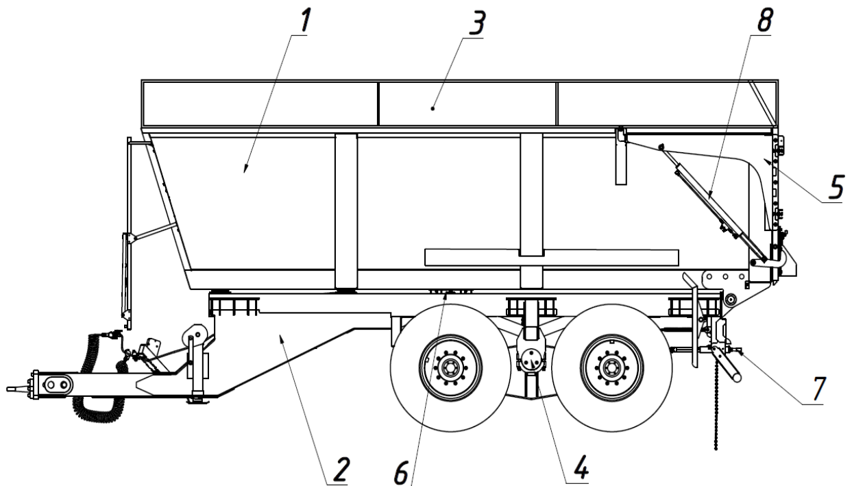
Рис. 1.1 Схема самосвального тракторного полуприцепа
